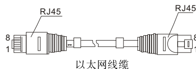
以太网线缆
