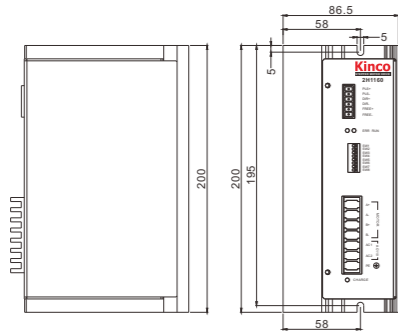
机械尺寸图 (单位: mm)
