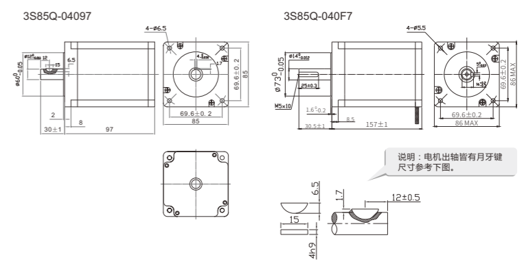
外形尺寸图 (单位: mm)
