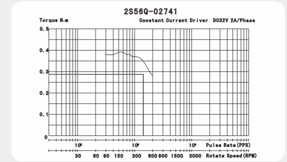
参考2S56Q-02741矩频曲线, 电机输出力矩符合要求。
